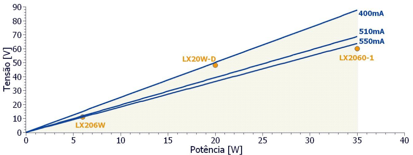
Figura 1 – Gráfico relação tensão x potência
