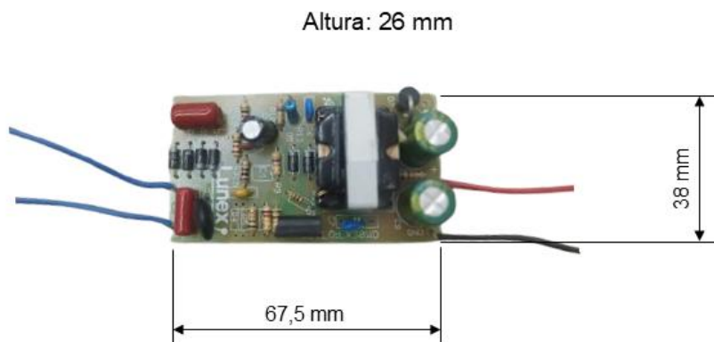
Figura 4 – Dimensões do produto.
