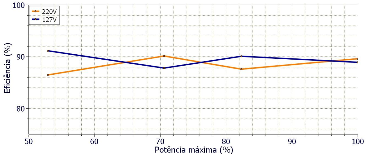
Figura 2 – Gráfico relação de carga x eficiência.
