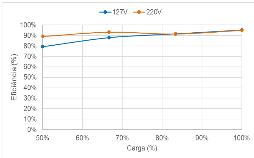
Figura 1 – Dados de Eficiência do produto LX1206 para diferentes potências.
