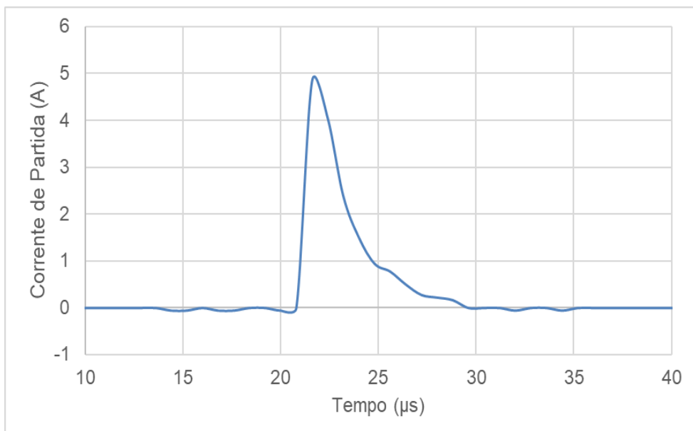
Figura 2 – Curva da corrente de partida da fonte LX1206.
