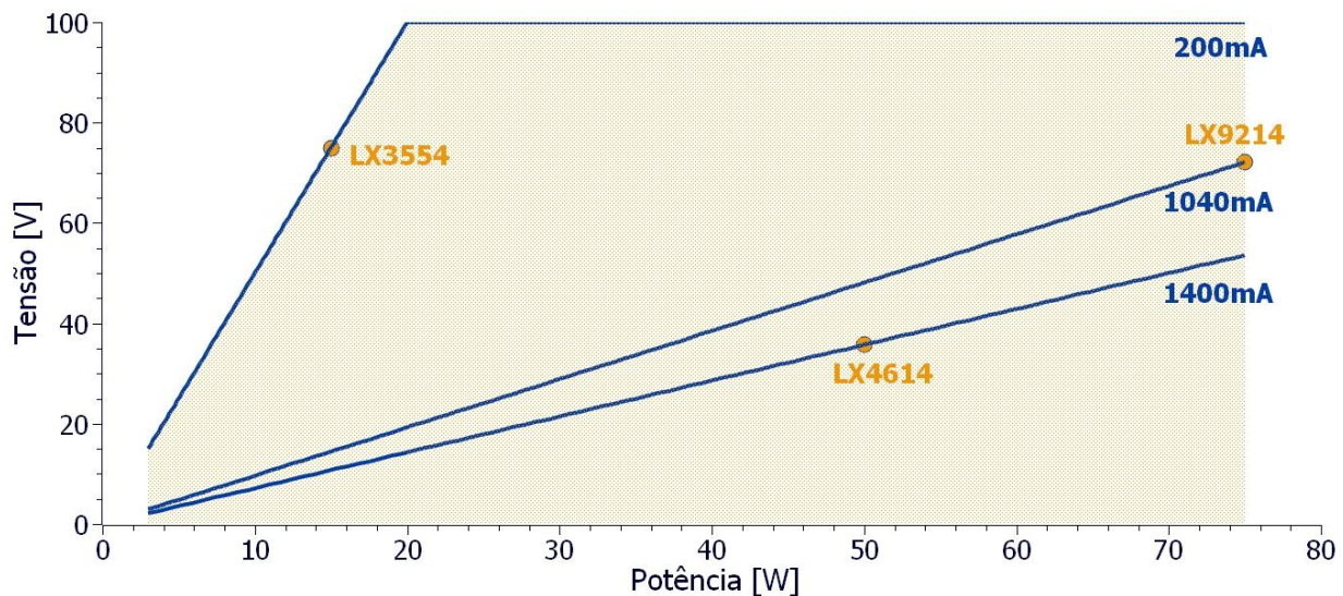
Figura 1 – Gráfico relação tensão x potência
