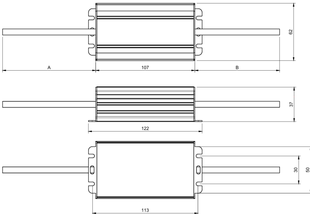
Figura 5 – Vistas do desenho mecânico.
