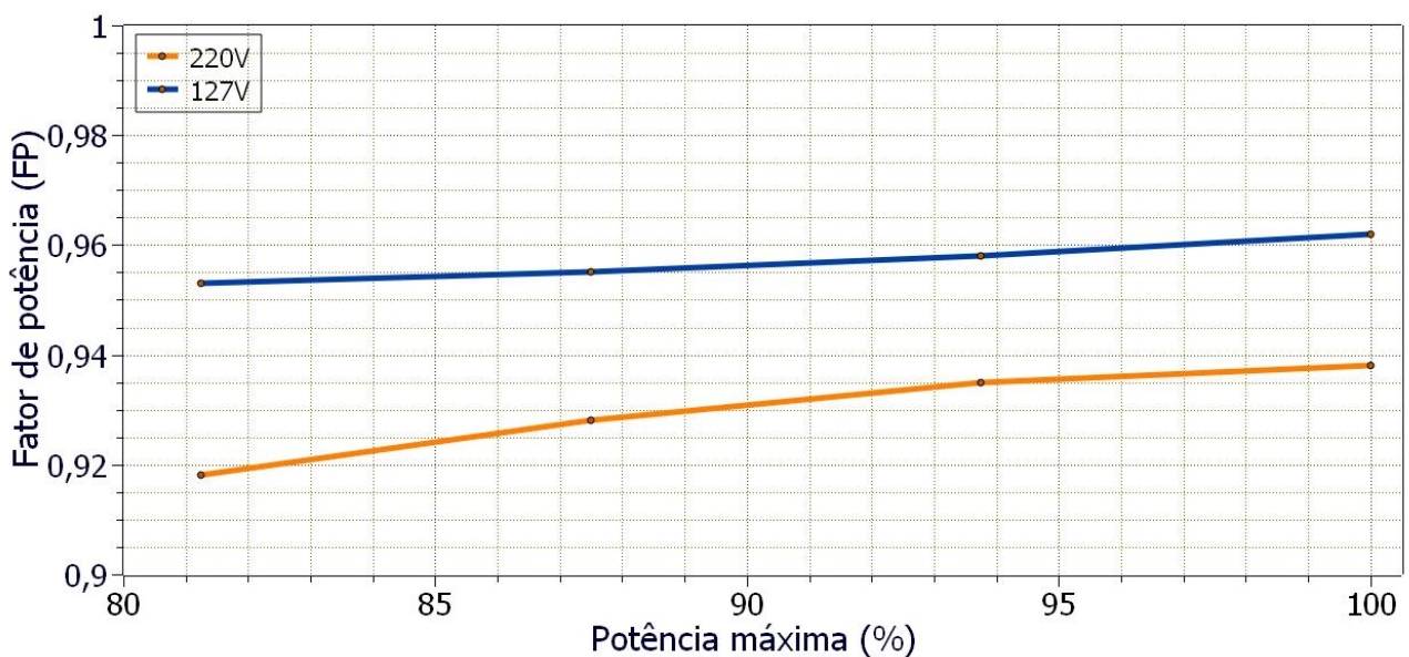
Figura 3 – Gráfico relação de carga x fator de potência
