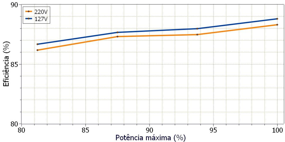
Figura 2 – Gráfico relação de carga x eficiência
