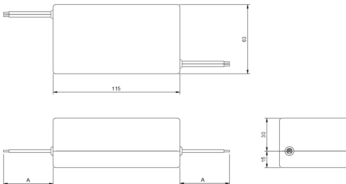
Figura 4 – Vistas do desenho mecânico.
