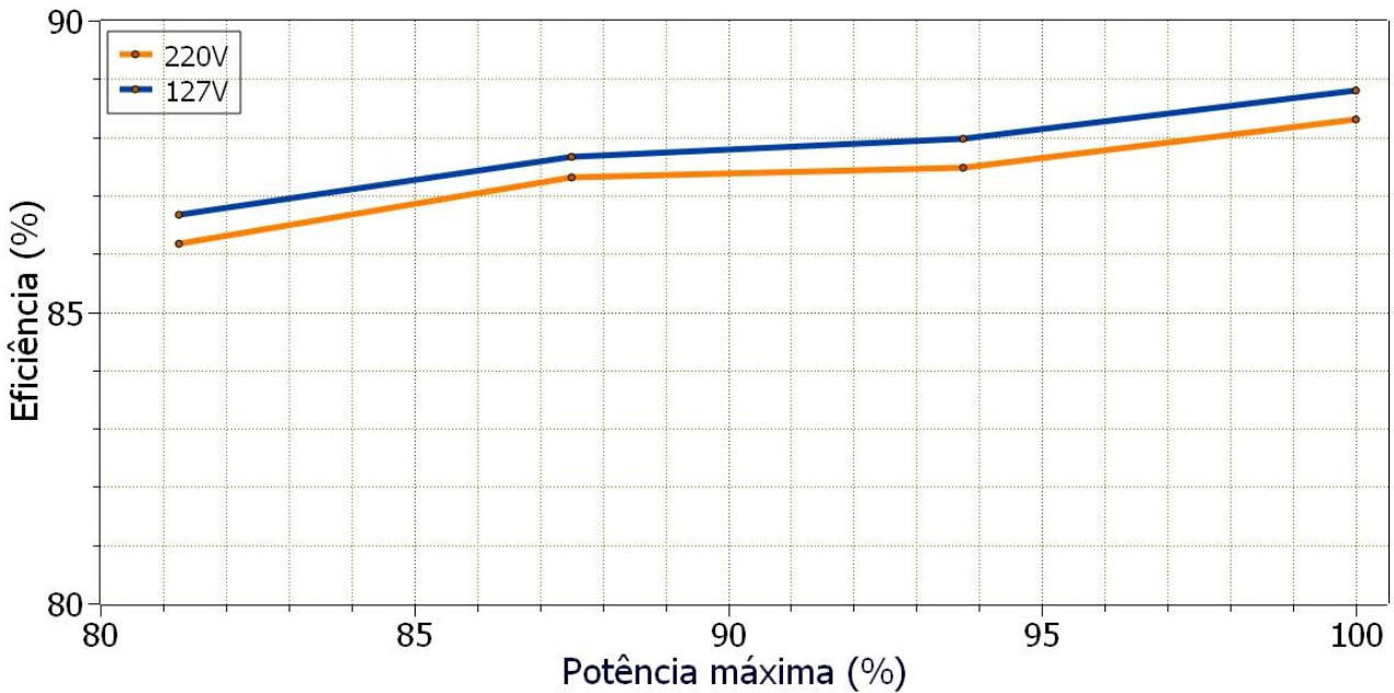
Figura 2 – Gráfico relação de carga x eficiência.
