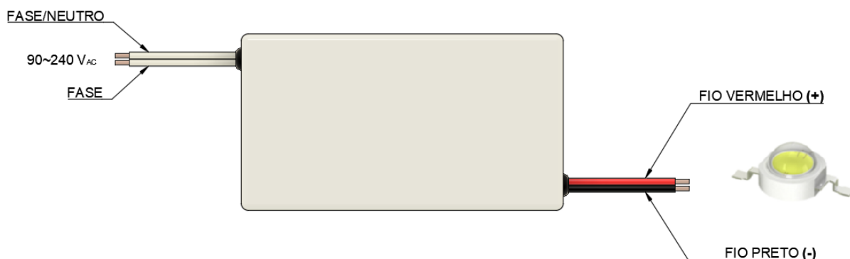
Figura 3 – Esquema de ligação.
