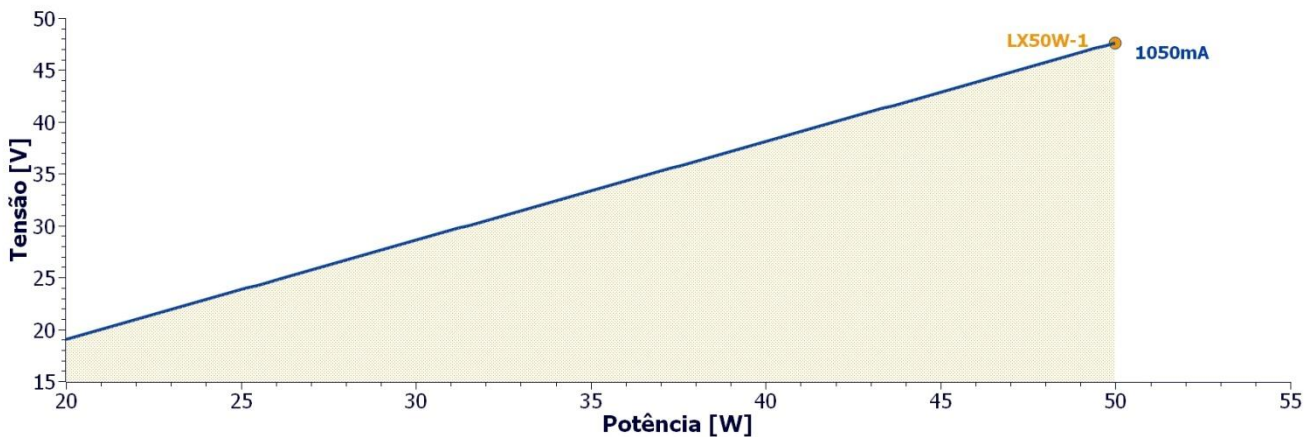
Figura 1 – Gráfico relação tensão x potência.
