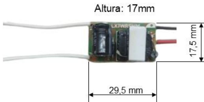
Figura 3 – Dimensões do produto.
