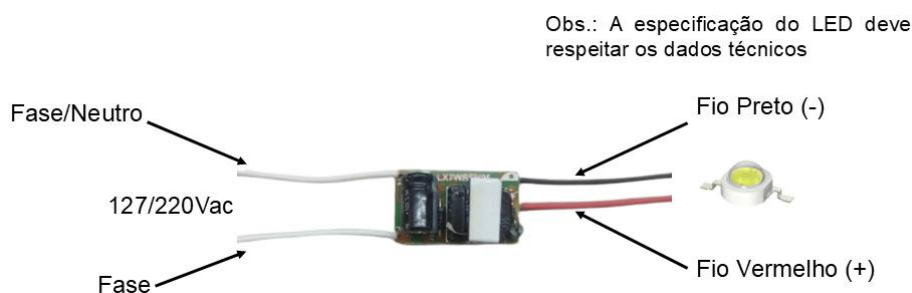
Figura 2 – Esquema de ligação.
