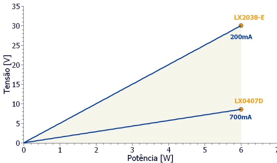
Figura 1 – Gráfico relação tensão x potência
